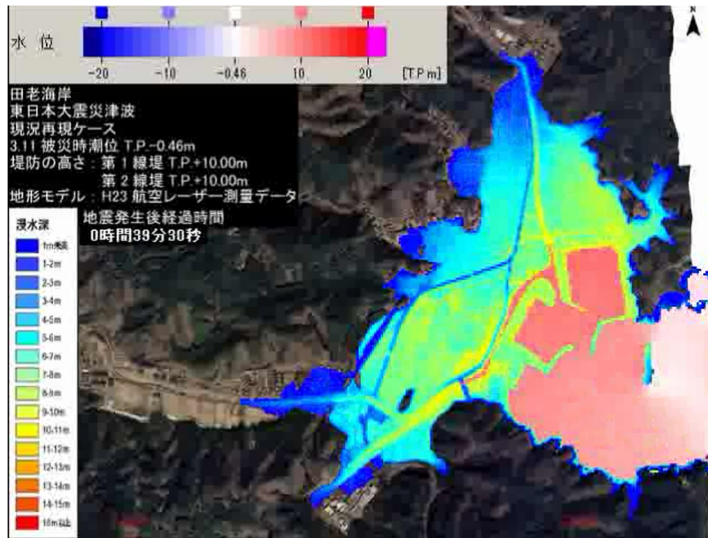
津波シミュレーション (再現計算)
